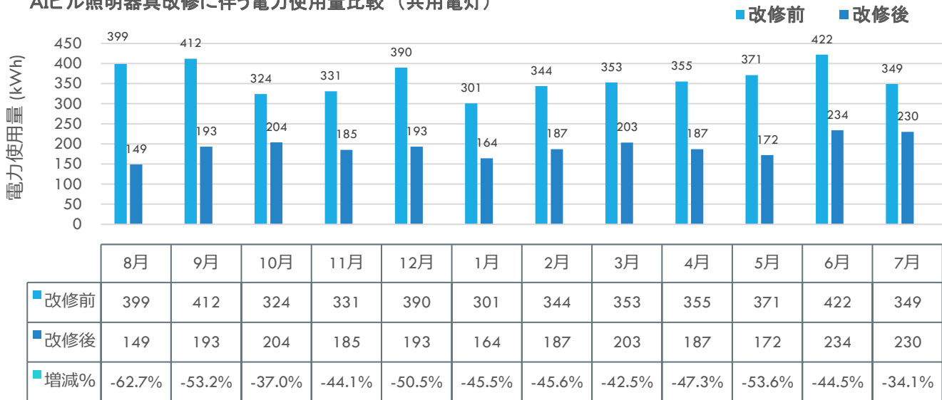
AIビル照明器具改修に伴う電力使用量比較（共用電灯）
